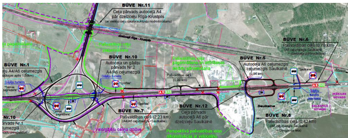
3.1.attēls. Izkopējums no AS Ceļuprojekts Tehniskā projekta "TEN autoceļu tīkla uzlabojumi, 2.projekts, 5.daļa, (A4 posms no km 18.9 līdz A6, A4/A6 ceļumezgls, A6 ceļumezgls Saulkalnē, autoceļam A6 "paralēlie" ceļi) risinājumu aktualizācija
