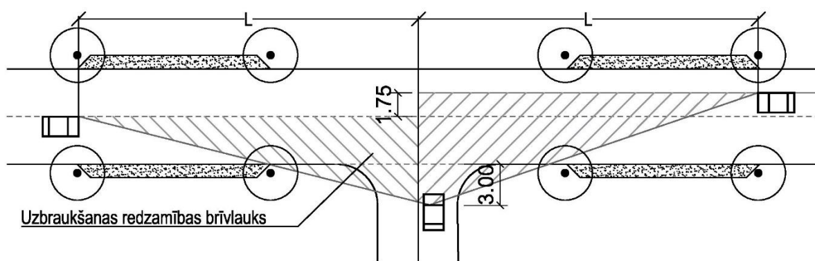
5.3..attēls. Uzbraukšanas redzamības brīvlauks
