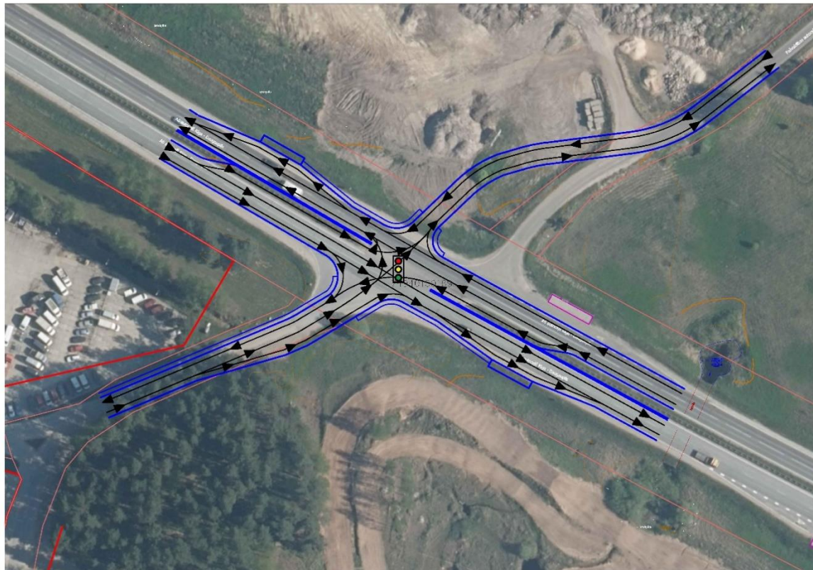
3.5.attēls. Elkšņu krustojums 1.variants
