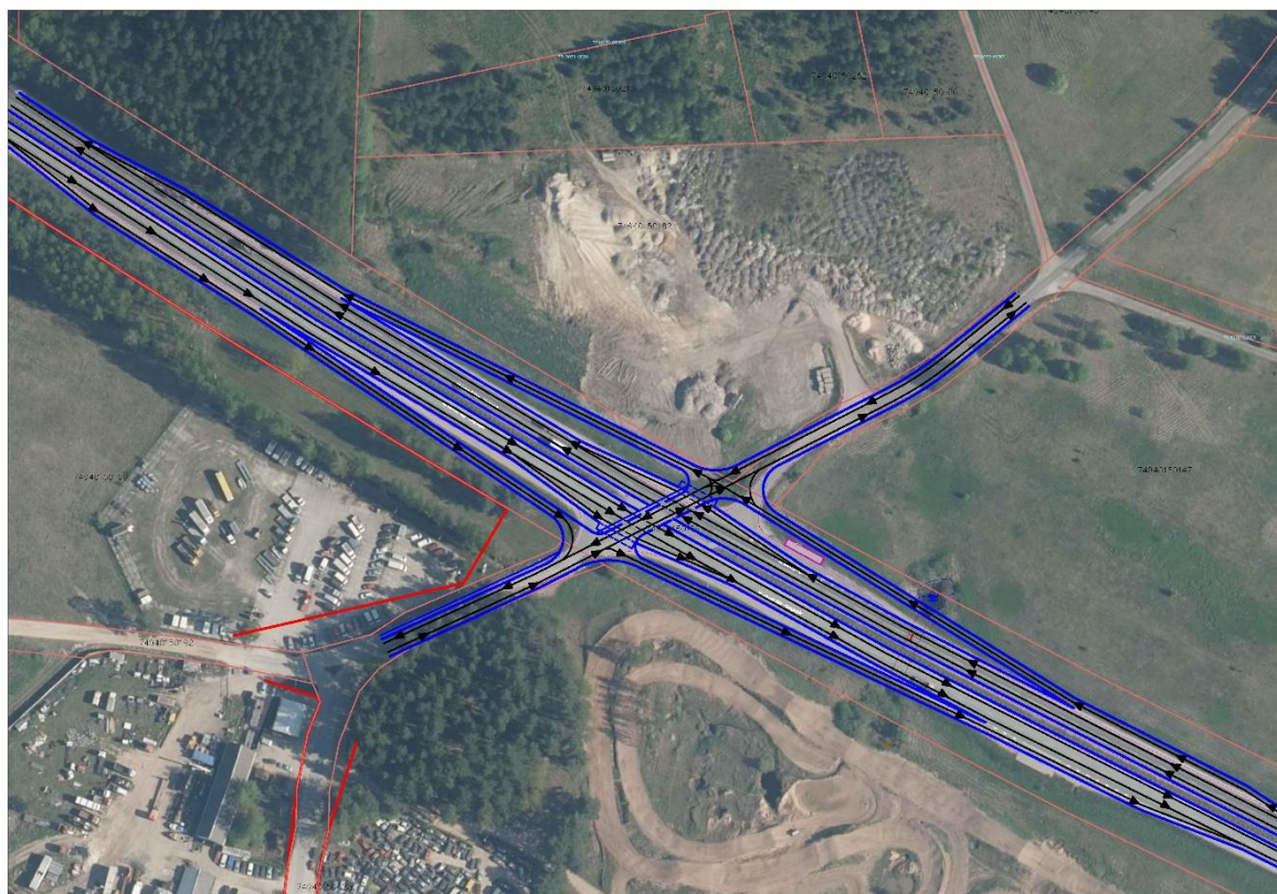
3.7. attēls. Elkšņu krustojums 3.variants
