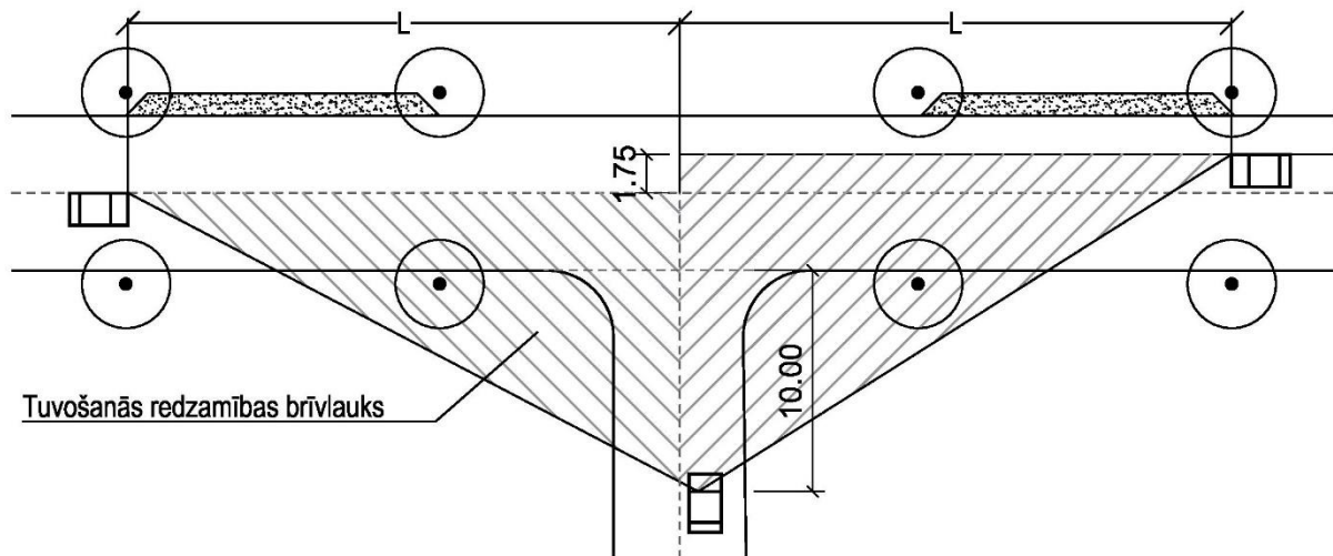
5.5.attēls. Tuvošanās redzamības brīvlauks
