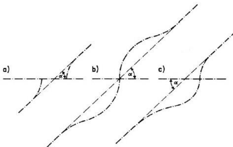
5.5.attēls. Pakārtotā ceļa ass līnijas pārveidošana, ja ir šaurs krustošanās leņķis. LVS 190-3
