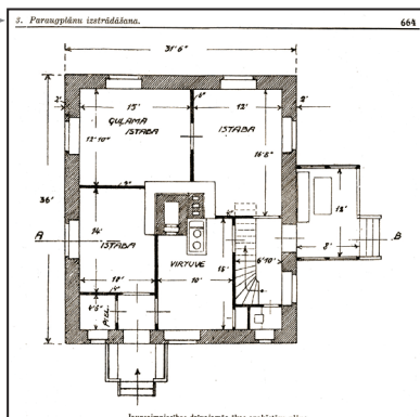
Jaunsaimniecības dzīvojamās ēkas apakšstāva plāns (Latvijas agrārā reforma., 664. lpp.)
